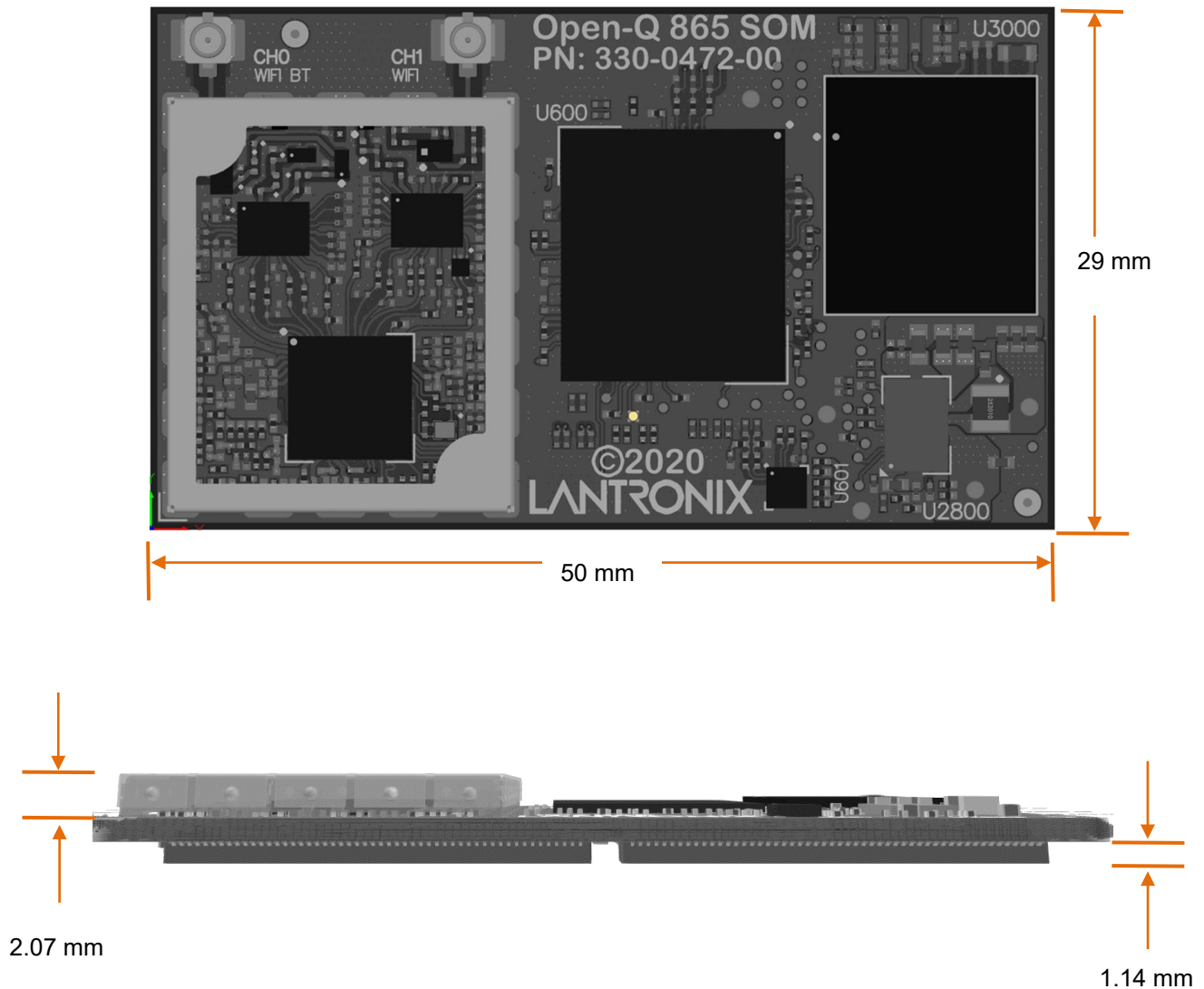
Figure 6: SOM Mechanical Outline (mm)
